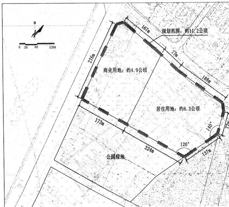
附图 2：用地红线图
